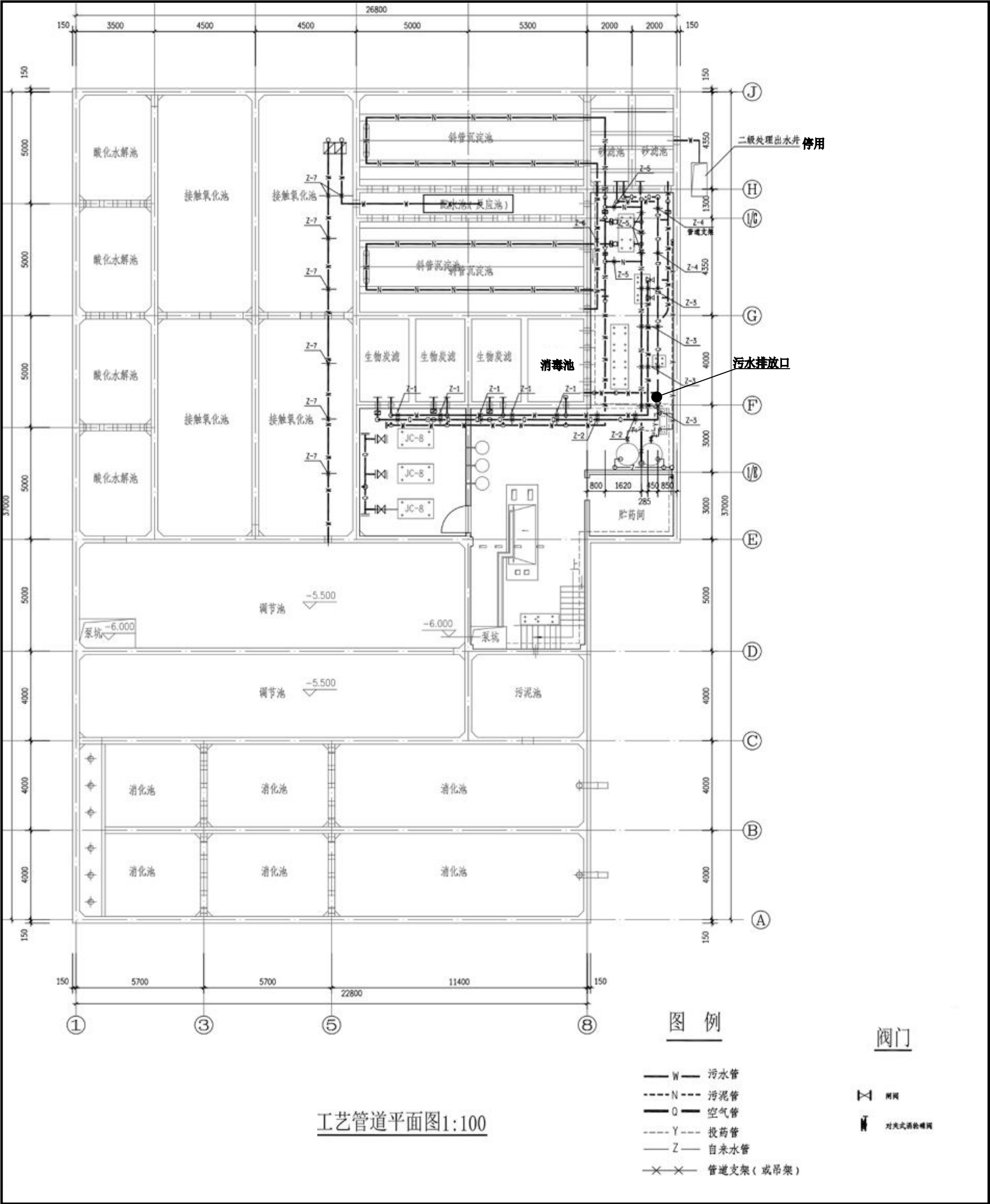
附件 5 污水处理站管线布置图
