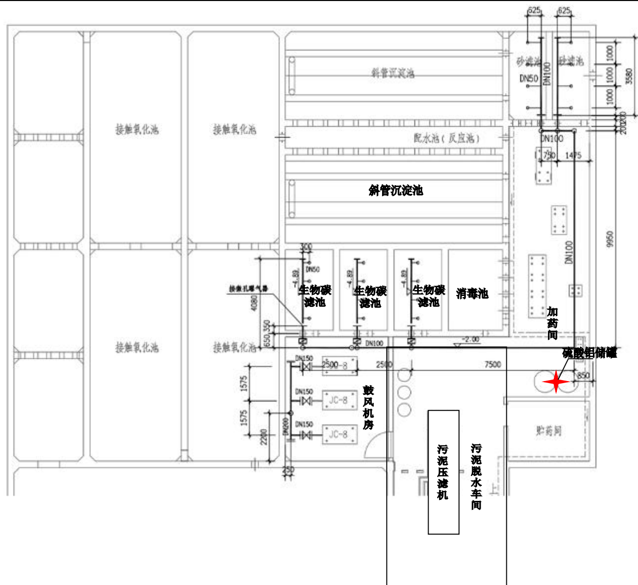
污水处理站地下平面图 (1: 100)
