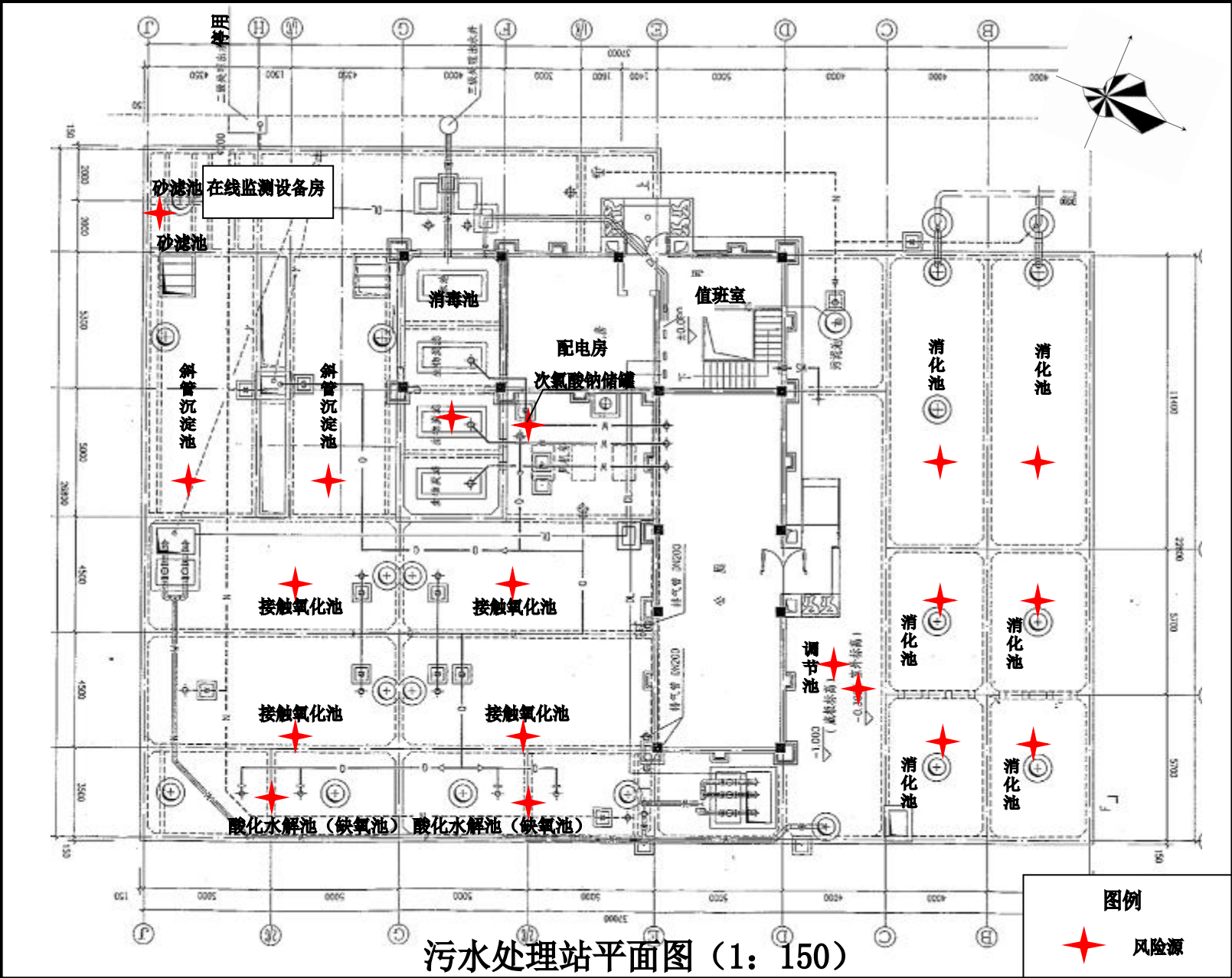
附件 4-1 污水处理站平面布置图
